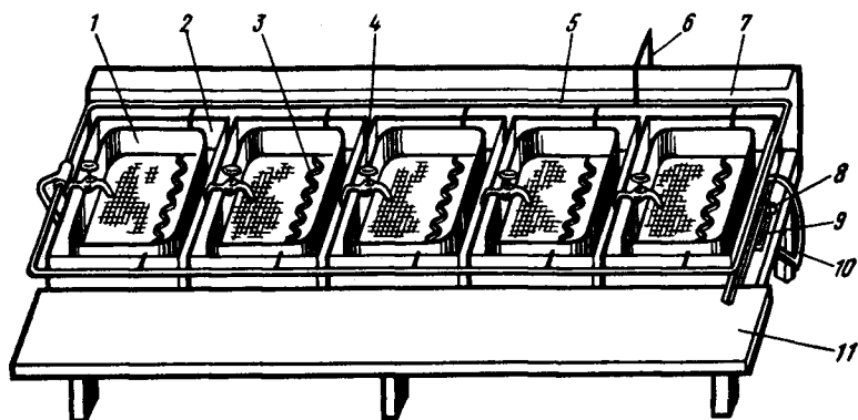
Рис. 47. Аппарат Ющенко (Ю-ИИ) для инкубации обесклеенной икры осетровых:
