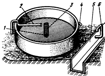
Рис. 62. Бассейн «Южаспрыбвода» (конструкция Бакгидропроекта): 1 — центральный сток; 2 — флейта; 3 — сетчатый цилиндр; 4 — аварийный сток; 5 — водосбросной желоб; 6 — регулятор водосброса
