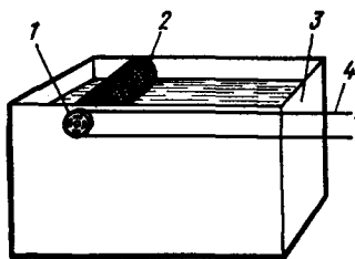
Рис. 54. Бак с барабаном для отмычки личинок хирономид от грунта: 1 — шкив; 2 — сетчатый барабан; 3 — корпус бака; 4 — приводной ремень
