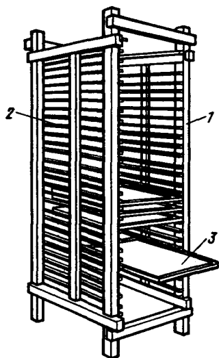
Рис. 53. Установка для разведения хирономид: 1 — стойка каркаса; 2 — опора для кювет; 3 — кюветы
