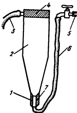
Рис. 43. Аппарат Вейса:
