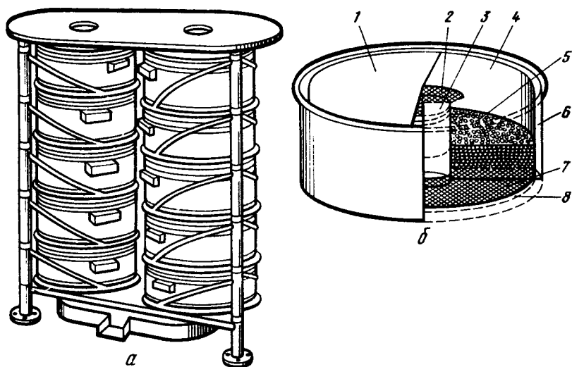
Рис. 41. Аппарат ИМ:
