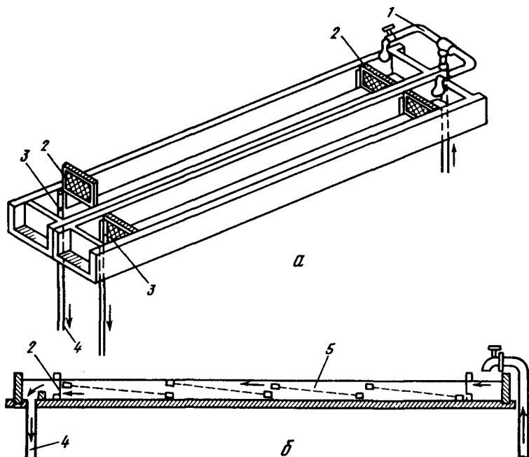
Рис. 39. Лотковый аппарат:
